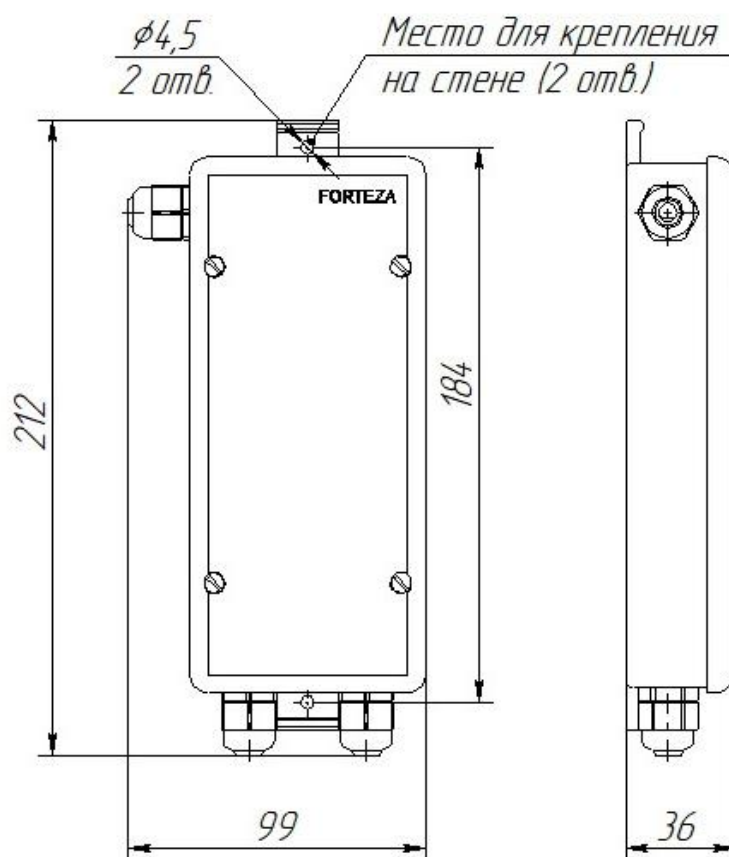
Рисунок 1 – Внешний вид коробки (стандартная комплектация)
