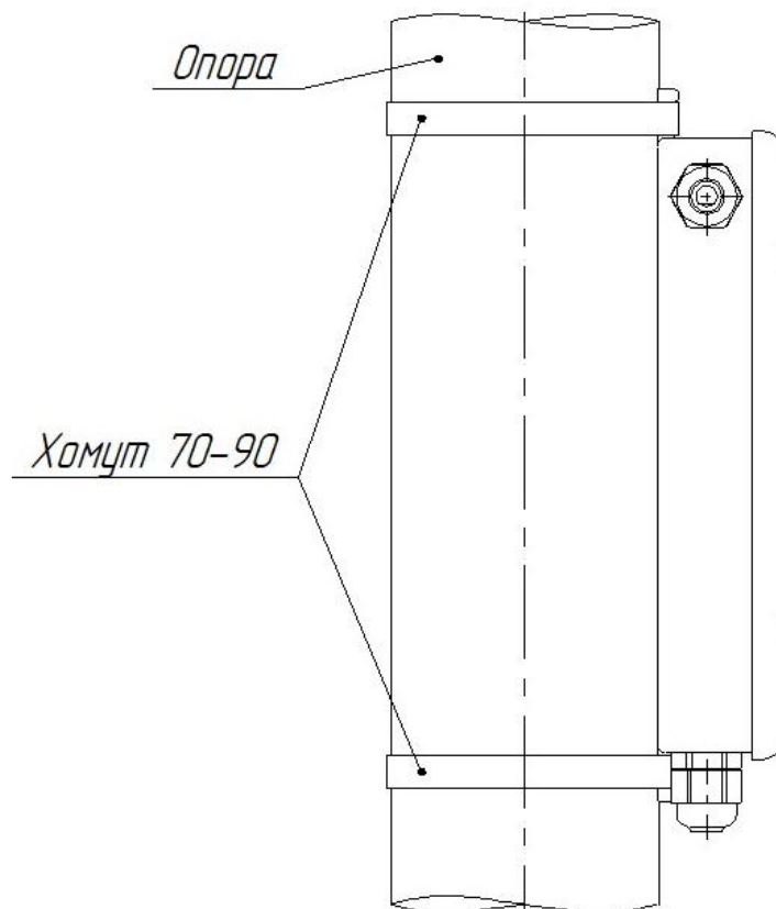
Рисунок 2 – Крепление коробки на опоре
